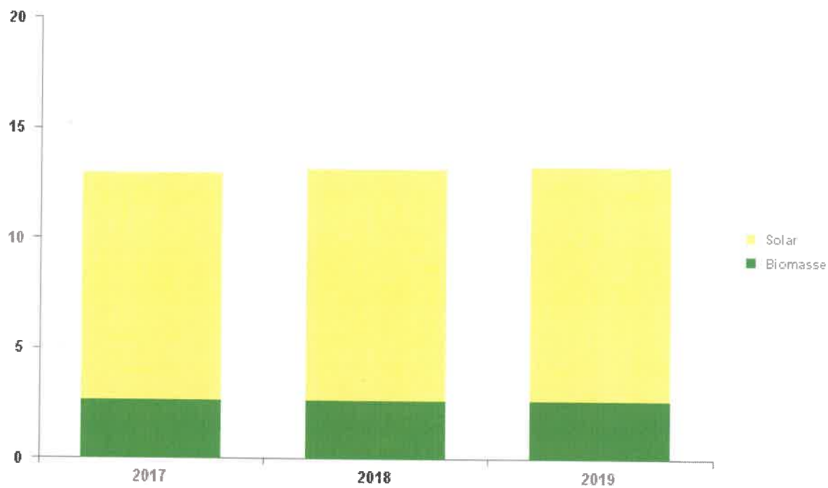
Installierte Einspeiserleistung in MW
